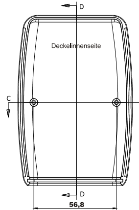
Deckelseite
