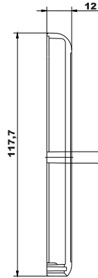
Schnitt D-D
