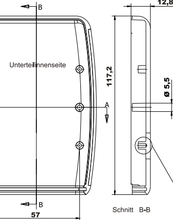
Unterteilöffnung
