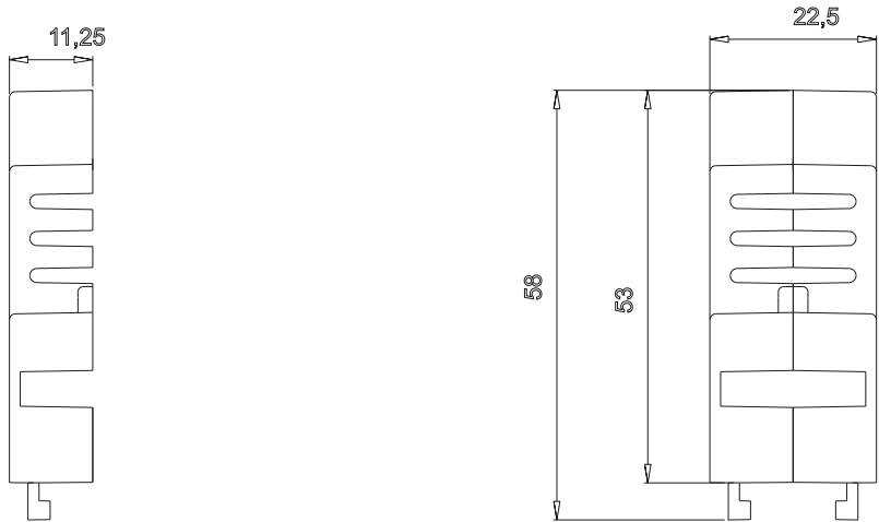
PCB Dimensions
